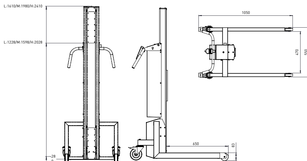
INOX 200 L/M/H - Leg 2
